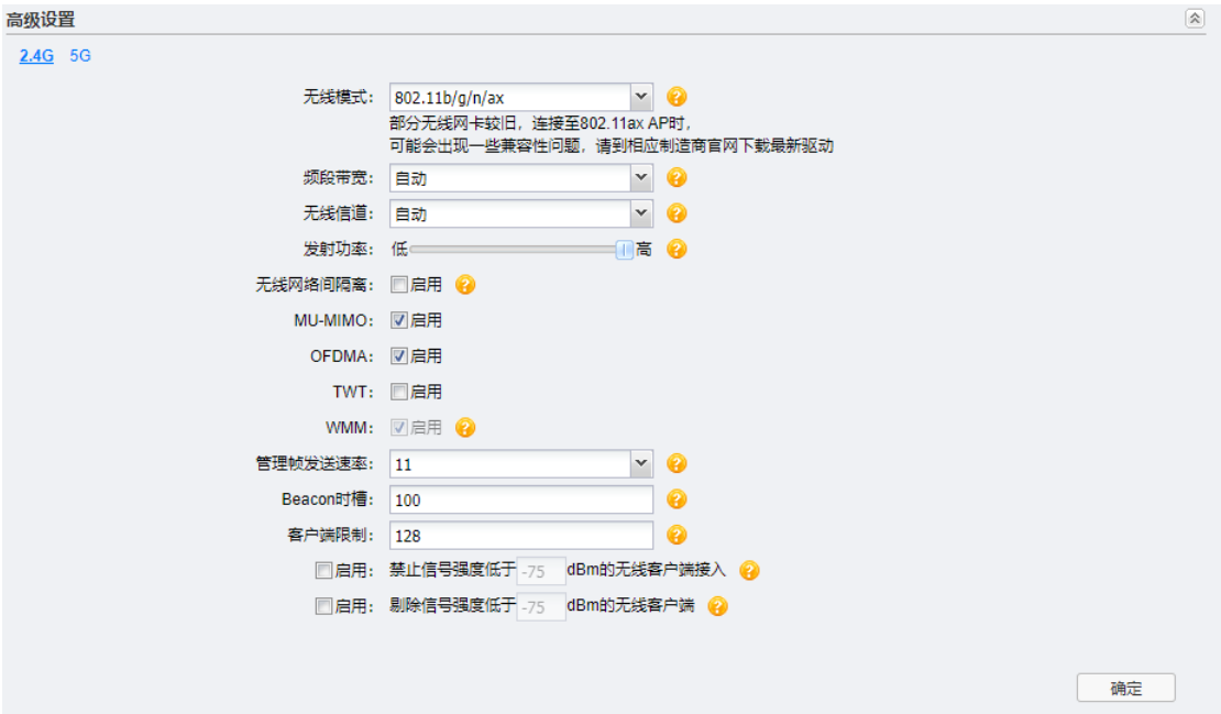
图 3-12 无线设置界面 - 高级设置区域
